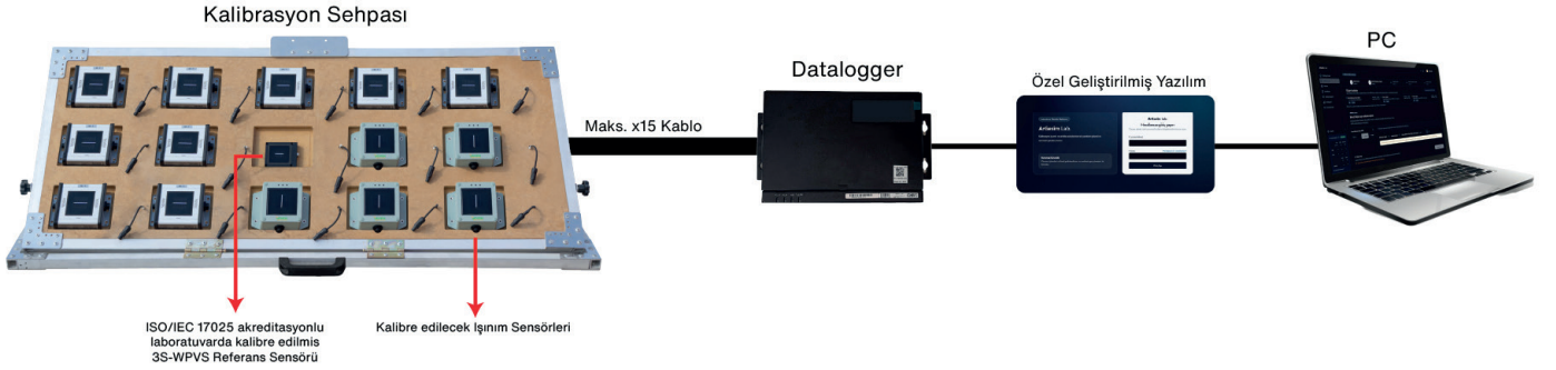
Görsel 1 - Işınım Sensörü Dış Ortam Kalibrasyon Ünitesi
