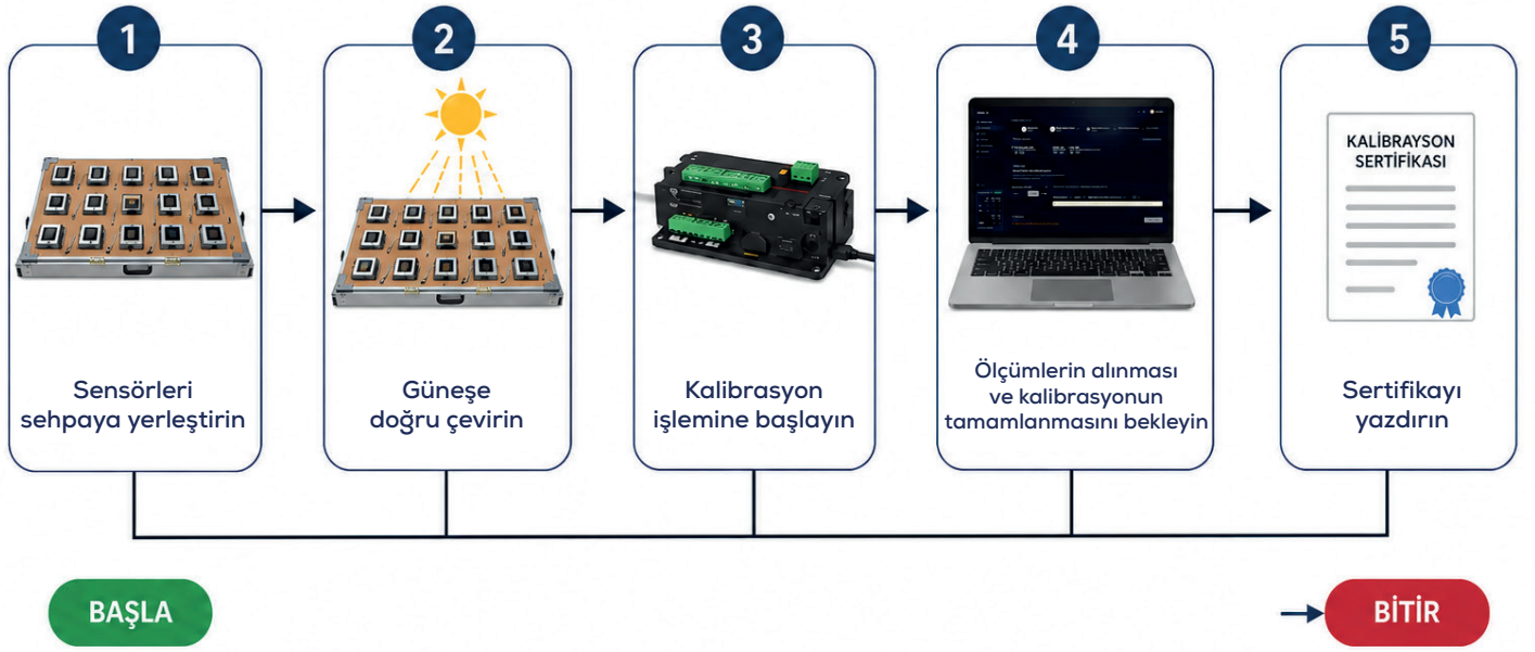
Görsel 9 - Kalibrasyon İşlemi Akış Şeması
