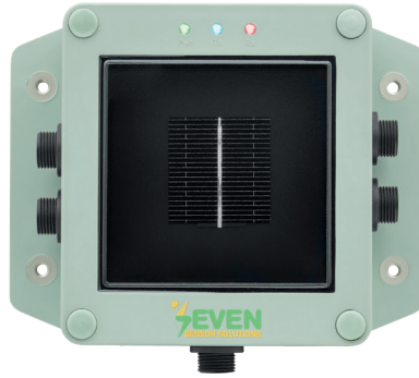
Görsel 3 - 3S-IS+ SEVEN Referans Işınım Sensörü
